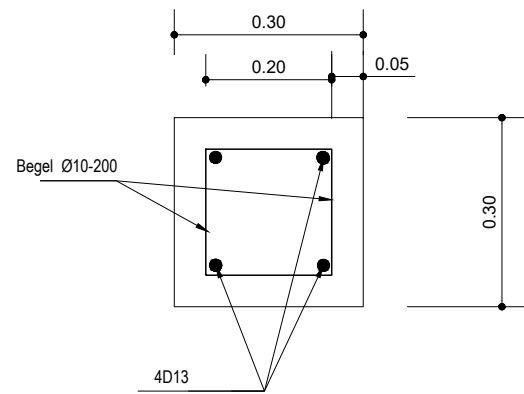
TIPIKAL PENULANGAN KOLOM DAN BALOK 30/30
