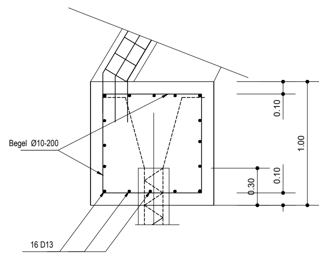
TIPIKAL PENULANGAN PONDASI 100/100
